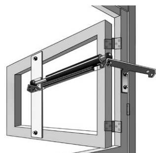
Установка на форточку с дополнительной планкой
