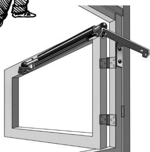
Установка на форточку
